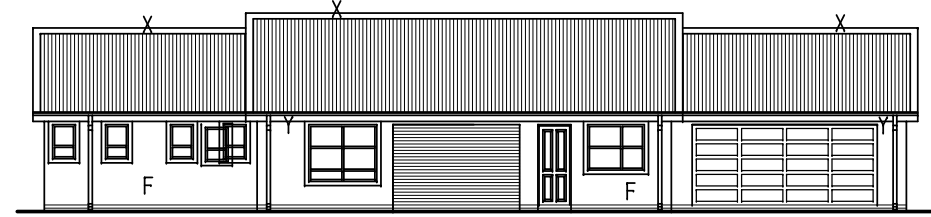
SUIDAANSIG skaal 1:200
