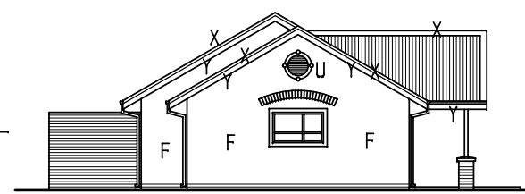
OOSAANSIG skaal 1:200
