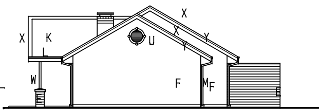
WESAANSIG skaal 1:200
